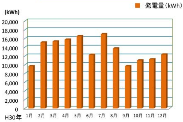
北杜9号、10号 発電実績
