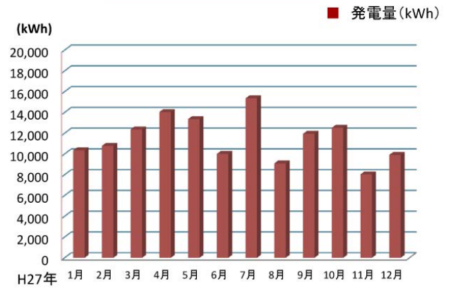
北杜3号、4号 発電実績
