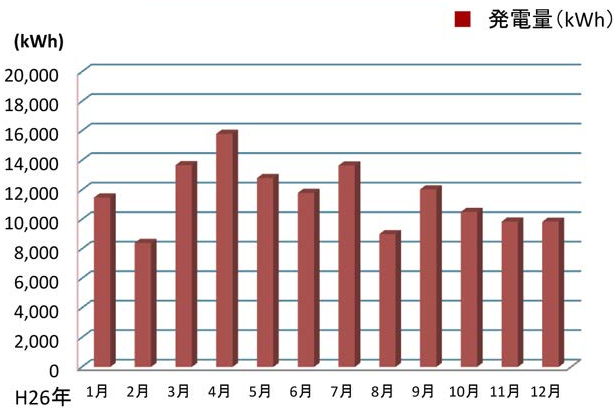
北杜3号、4号 発電実績
