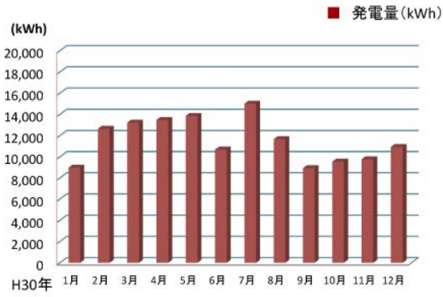
北杜3号、4号 発電実績
