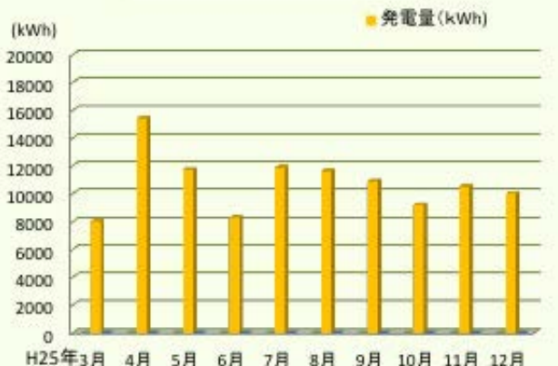
北杜1号、2号 発電実績
