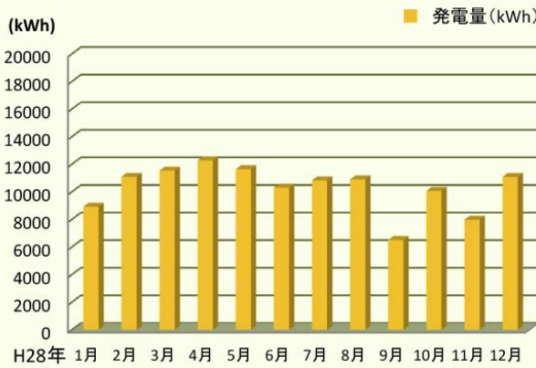
北杜1号、2号 発電実績
